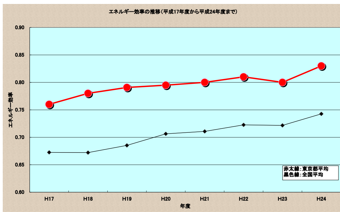
図. 東京都における地域冷暖房のエネルギー効率の推移
